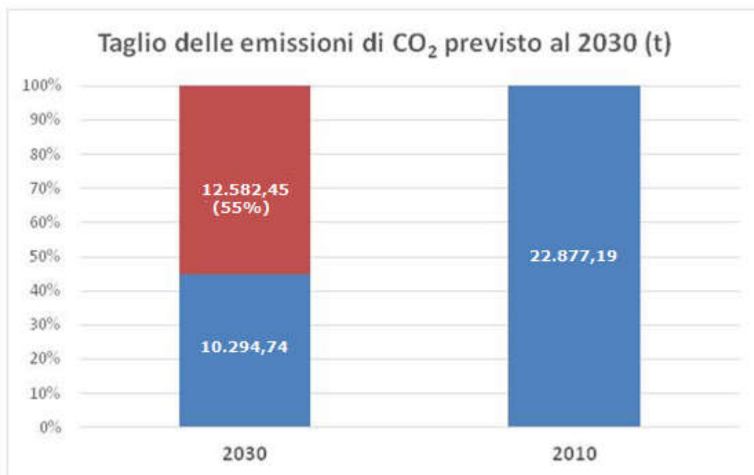
Figura 3.20: Emissioni di CO 2 nel Comune di San Pancrazio Salentino nell'anno di riferimento 2010 ed obiettivo minimo di riduzione del 55% delle stesse entro il 2030 (in rosso la quantità corrispondente)
