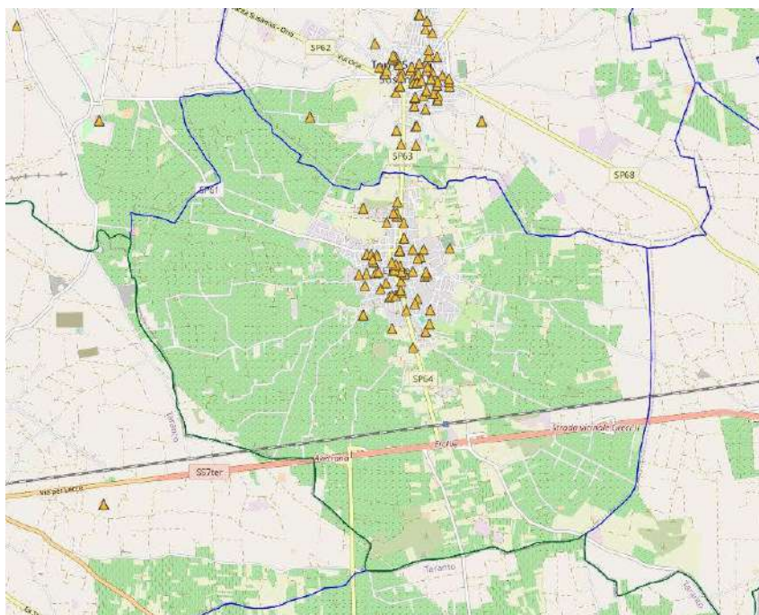
Figura 3.16: Installazioni di solare termico localizzate nel Comune di Erchie (Fonte: GSE - portale Atlaimpianti)
