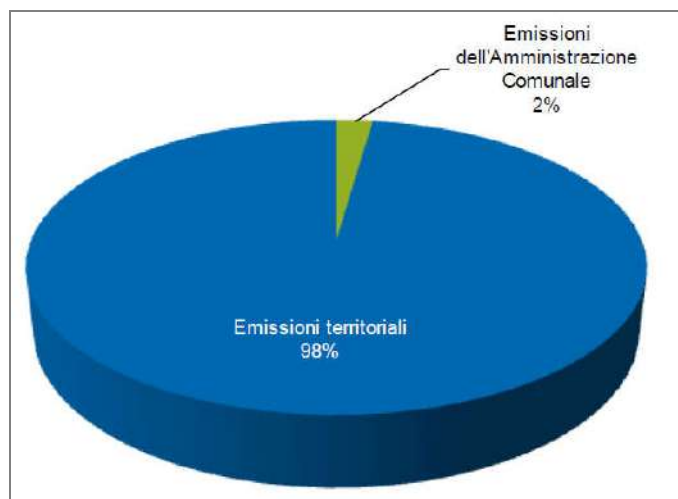
Figura 3.9: Ripartizione delle emissioni di CO 2 fra quelle di competenza territoriale e quelle di competenza comunale
