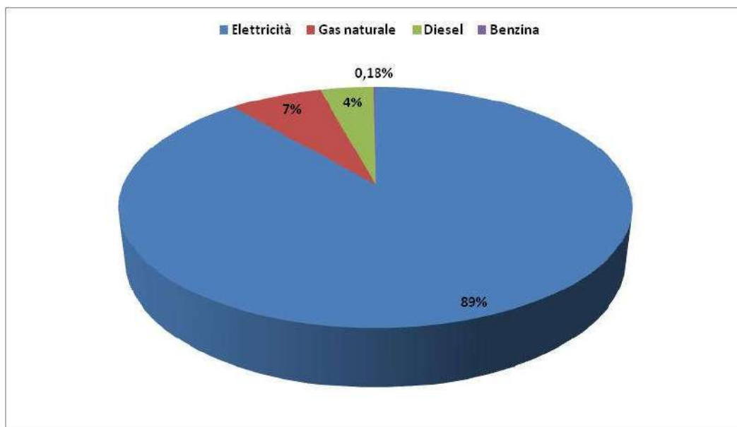
Figura 3.11: Ripartizione delle emissioni comunali di CO 2 per vettore energetico
