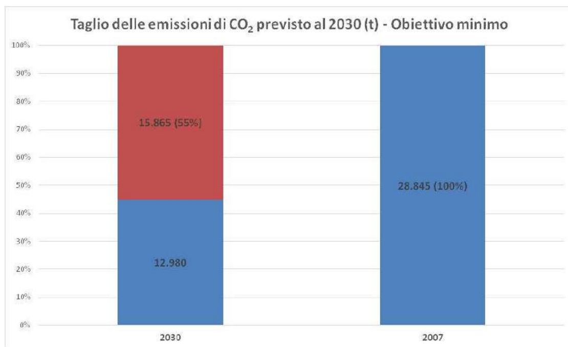
Figura 3.14: Emissioni di CO 2 nel Comune di Erchie nell'anno di riferimento 2007 ed obiettivo minimo di riduzione del 55% delle stesse entro il 2030 (in rosso la quantità corrispondente)
