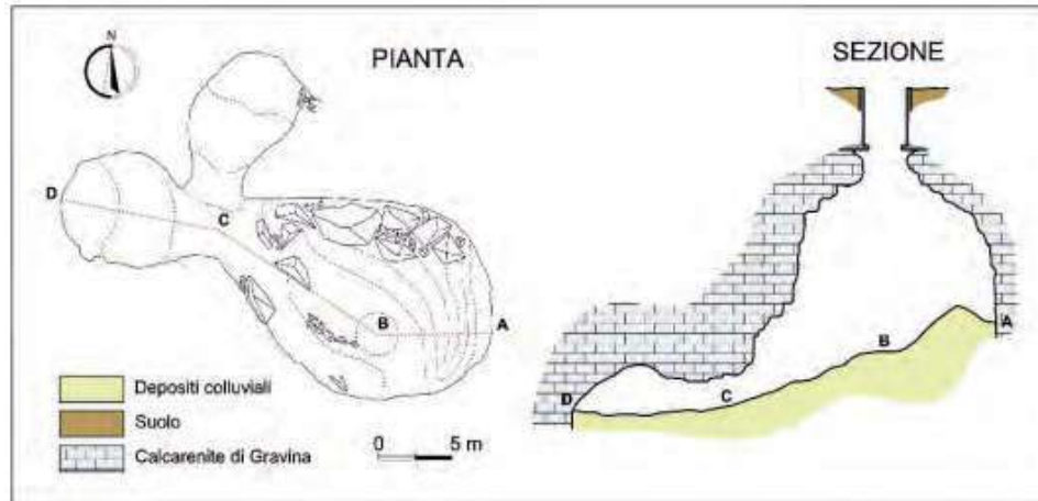
Figura 5.20: Pianta e sezione di una Vora (da AA.VV. 2008)
