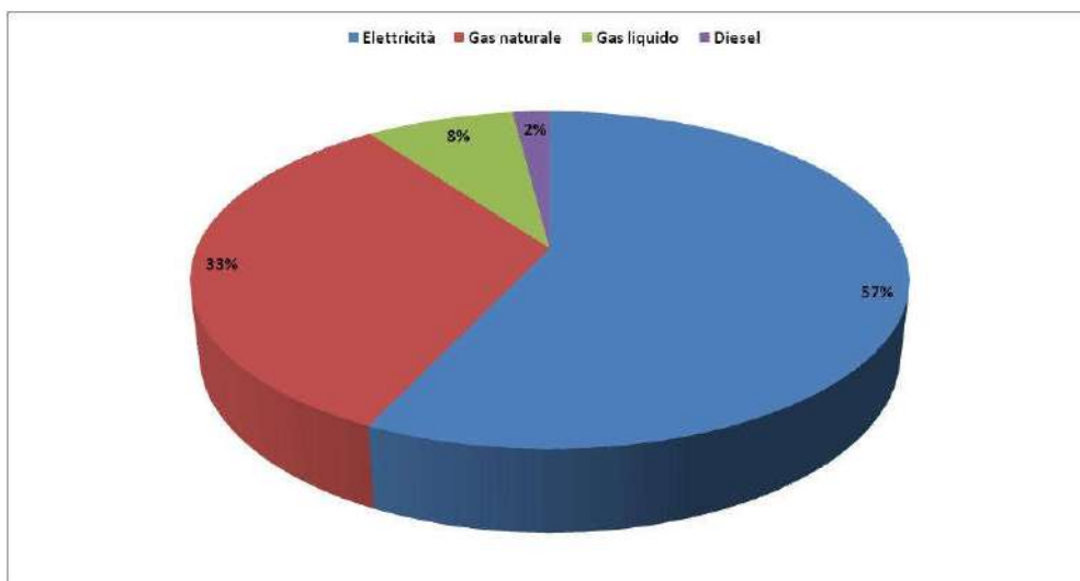
Figura 3.7: Ripartizione delle emissioni di CO 2 per vettore energetico per la categoria edifici, attrezzature e impianti
