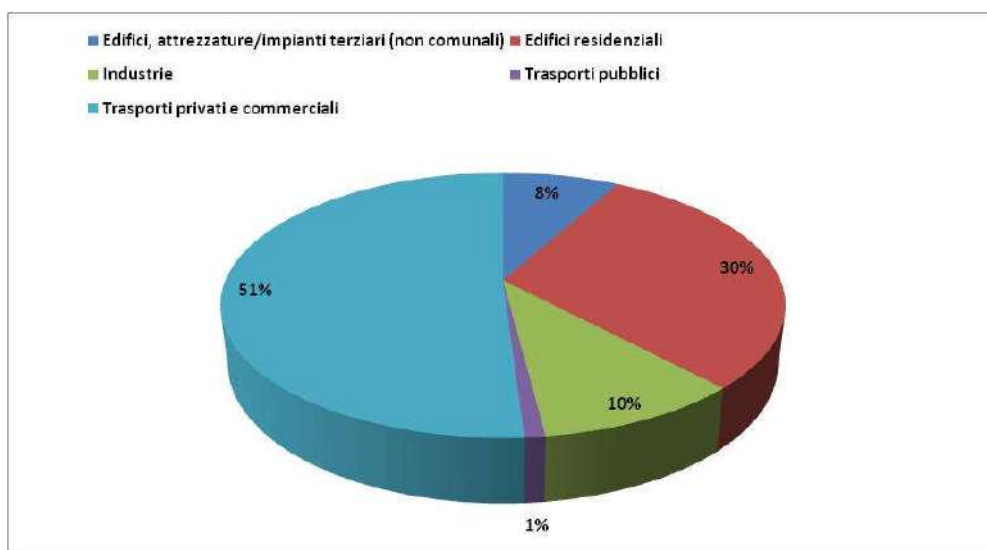
Figura 3.12: Ripartizione delle emissioni territoriali di CO 2 per categoria
