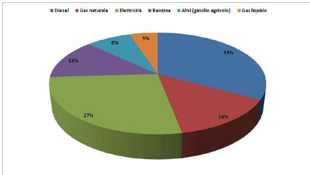
Figura 3.6: Ripartizione delle emissioni totali di CO 2 per vettore energetico
