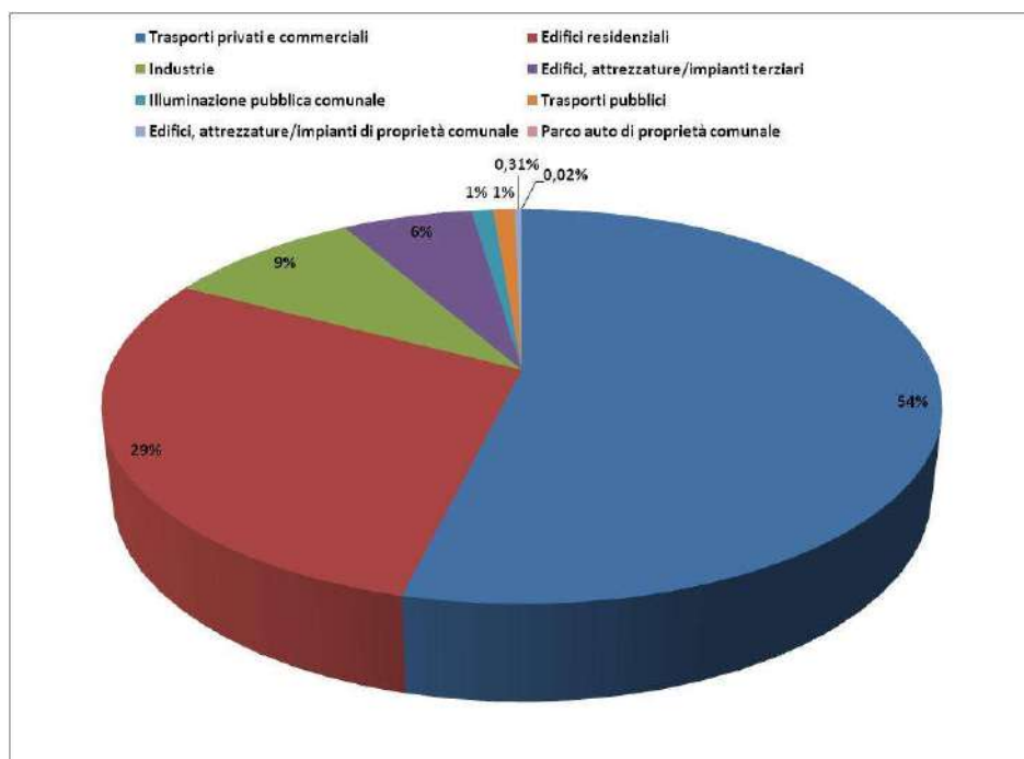
Figura 3.3: Ripartizione dei consumi energetici totali per categoria
