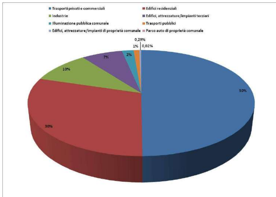
Figura 3.4: Ripartizione delle emissioni totali di CO 2 per categoria
