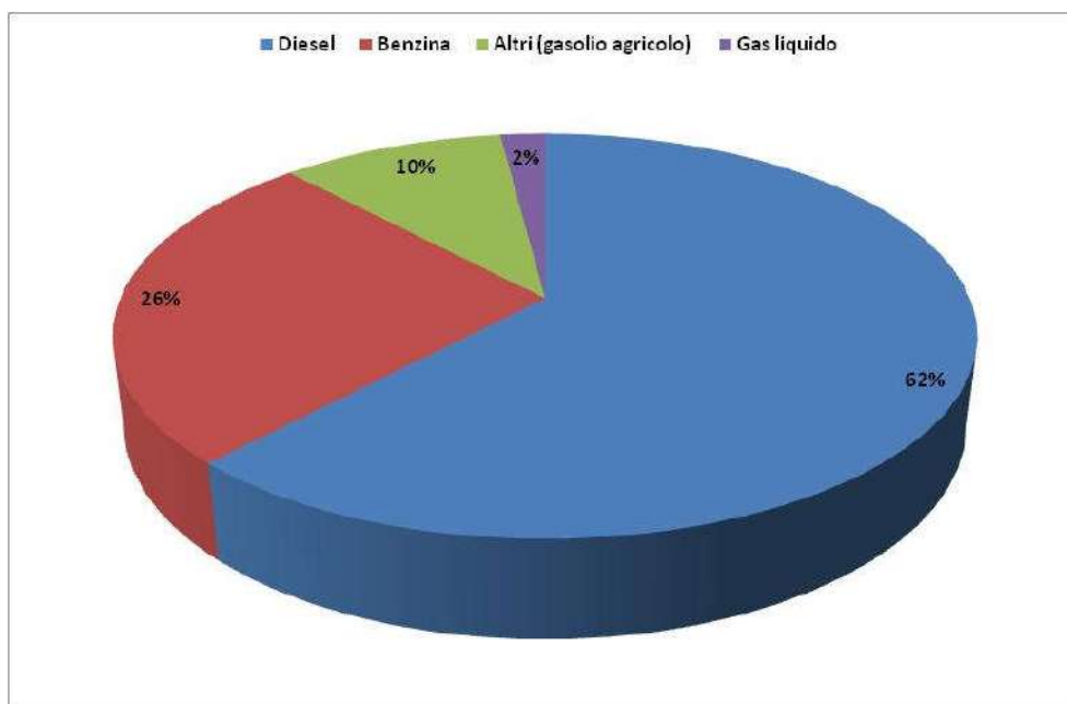
Figura 3.8: Ripartizione delle emissioni di CO 2 per vettore energetico per la categoria trasporti
