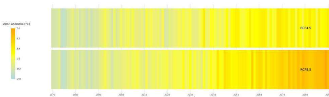
Figura 5.17: Proiezioni future fino al 2100 – Anomalie dell'indice TMEAN
