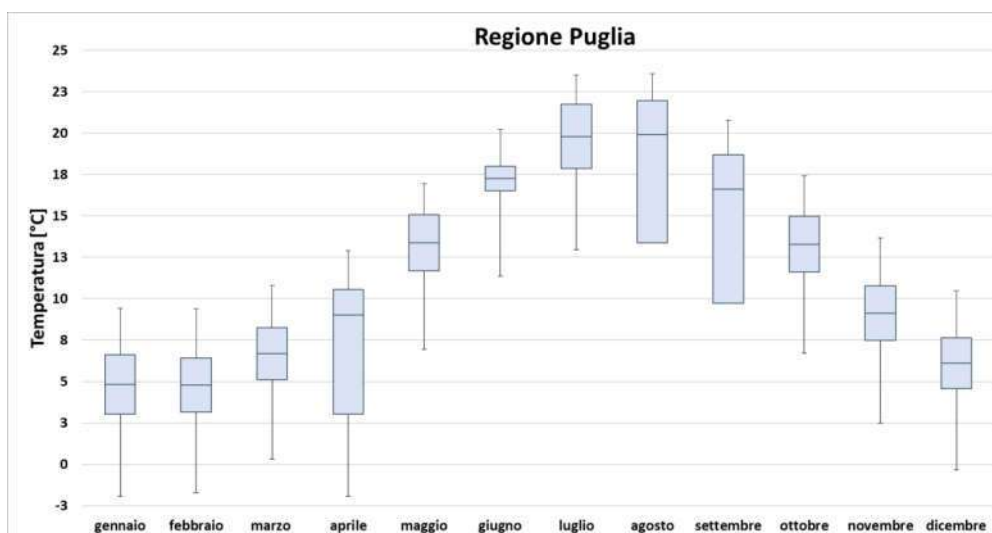
Figura 5.8: Andamento delle temperature medie minime spaziali (minime e massime spaziali assolute) per l'anno storico (fonte: elaborazione SRACC su dati della Protezione Civile)
